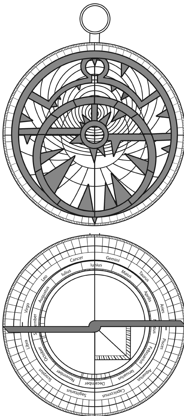
Obr. 3 – Možná podoba astrolábu podle nejstarších středověkých latinských textů; nahore přední strana a rete (tmavší), dole zadní strana s alhidádou (tmavší)
