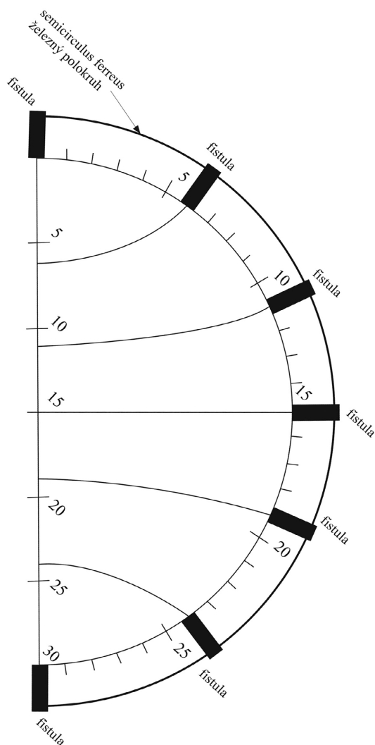
Obr. 2 – Gerbertova pozorovací hemisféra
