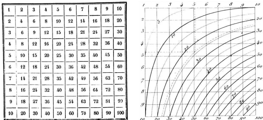
Obr. 28: Pouchetova pythagorejská tabulka a isočáry xy = 5k , k = 0, 1, \dots, 19 (1795).
