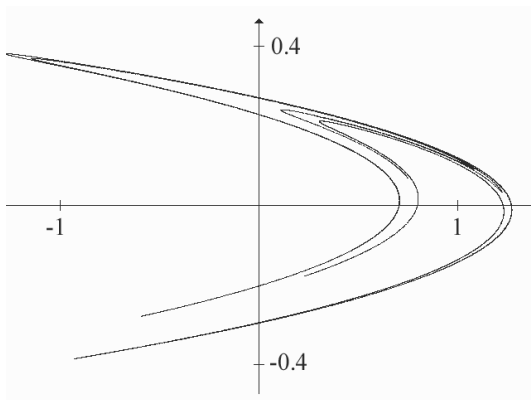
Obr. 3. Hénonův podivný atraktor zobrazení T v oblasti (-1.3, 1.3) \times (-0.4, 0.4) .
