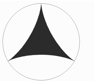
Obr. 4. Černě je obarvena oblast ohraničená Steinerovou hypocykloidou uvnitř kružnice o poloměru 3/4 .
