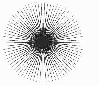
Obr. 5. Plocha složená z mnoha dlouhých a úzkých trojúhelníků.
