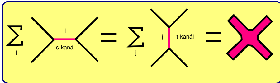
Obr. 1. Dva druhy Feynmanových diagramů ( s, t -kanály) lze přepsat jako Feynmanův diagram pro strunu (vpravo), a proto jsou si rovny.
