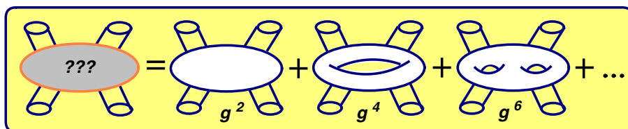
Obr. 2. Amplituda elastického rozptylu dvou uzavřených strun jako mocninový rozvoj ve vazebné konstantě.
