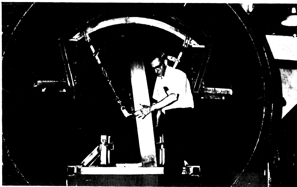
Profesor Weber u marylandského disku detektoru gravitačních vln (k článku V. Marvanové). Detektor gravitačních vln v Braginského laboratoři v Moskvě (k článku V. Marvanové).
