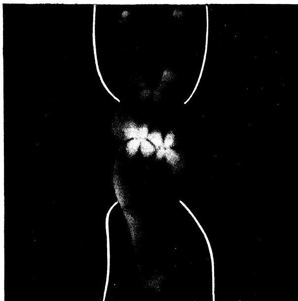
Obr. 9. Izochromatické křivky na modelu řezu horní a dolní čelisti.
