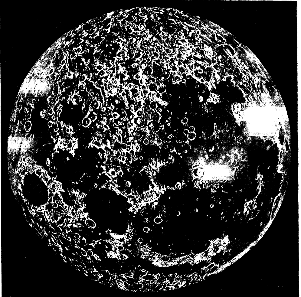
Obr. 2. Andělova figurální mapa Měsíce (převzato z knihy Vl. Guth, F. Link, J. M. Mohr, B. Šternberk, Astronomie I , NČSAV, Praha 1954).
