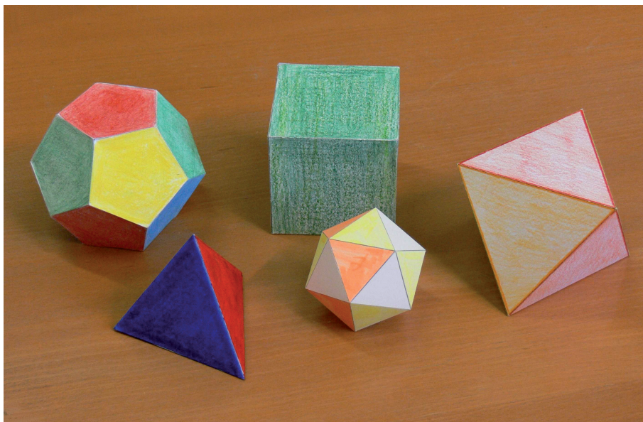
Obrázek I: Pravidelné mnohostěny
