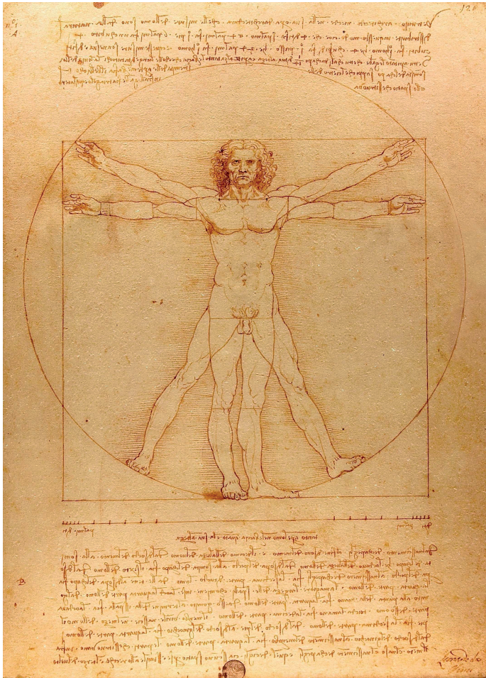
Obrázek III: Vitruviánský muž
