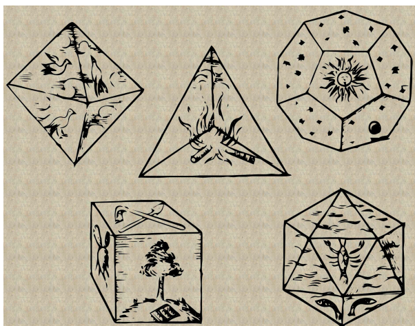
Obrázek II: Pravidelné mnohostěny jako symboly živlů
