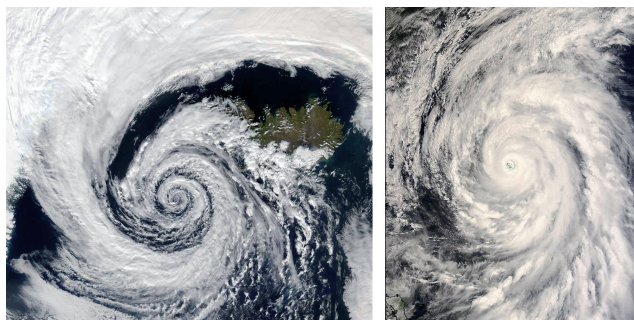
Obrázek XII: Zleva: Oko hurikánu, tlaková níže nad Islandem
