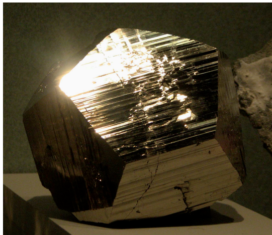
Obrázek XI: Pyrit
