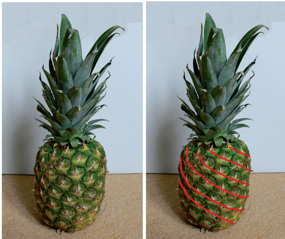
Obrázek XVI: Parastichy na povrchu ananasu
