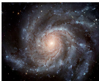
Obrázek XIII: Galaxie M101
