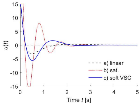
Fig. 5. Control input.
