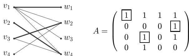
Obr. 4. Maximální párování v bipartitním grafu (vlevo); matice grafu s vyznačenými jedničkami, které odpovídají zvolenému párování (vpravo)
