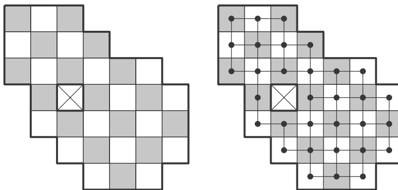
Obr. 2. Obrazec vlevo lze pokrýt dominy, právě když v grafu vpravo existuje perfektní párování
