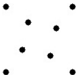
Obr. 4: Uspořádání 8 bodů v rovině, které neobsahuje konvexní pětiúhelník.
