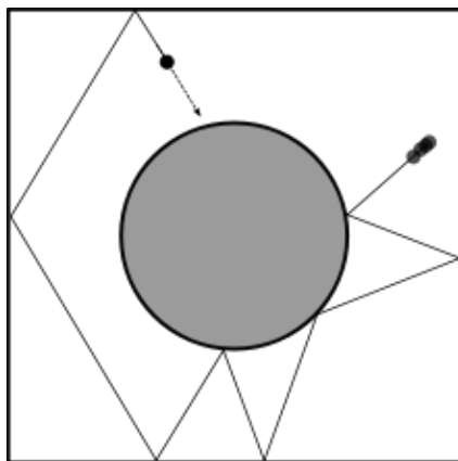
Obr. 3. Sinajův kulečnick (nakreslil Georg Stamatiou)
