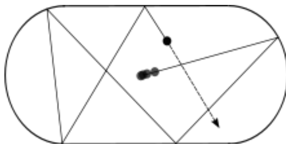
Obr. 4. Bunimovičův kulečnick (nakreslil Georg Stamatiou)
