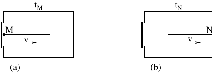
Obr. 13. Zavření dveří ( M ) a náraz na protější stěnu ( N ).
