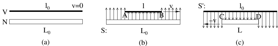
Obr. 1. Vlak a nádraží.
