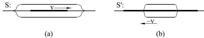
Obr. 2. Vlak a kolejiště.
