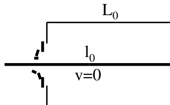
Obr. 14. Zastavená tyč se do stodoly nevejde.
