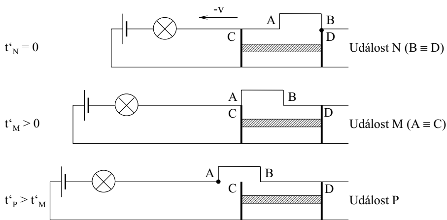
Obr. 19. V události P dorazila zpráva o události N do bodu A .
