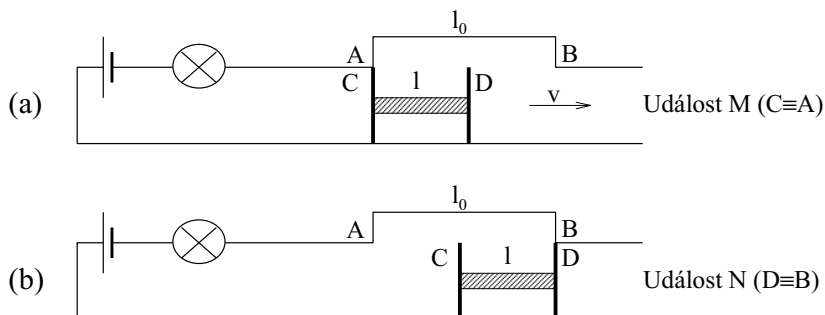
Obr. 17. Kontakt je po dobu t_N - t_M přerušen.
