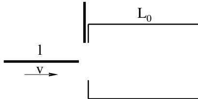
Obr. 12. Zkrácená pohybující se tyč vletí do kůlny.
