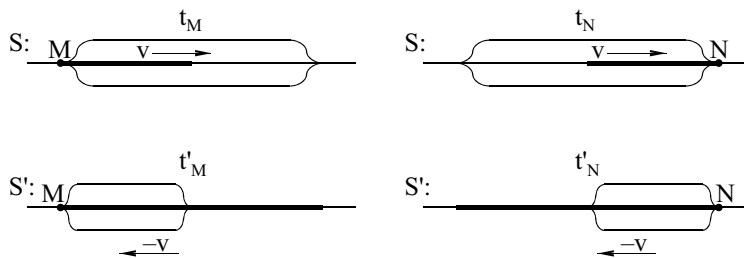
Obr. 3. Vjezd konce a výjezd začátku vlaku.
