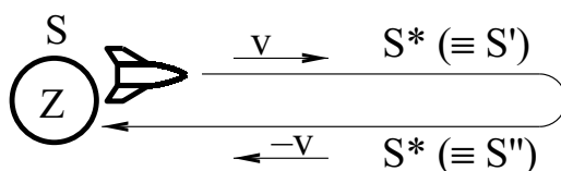
Obr. 10. Paradox dvojčat.
