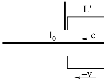
Obr. 15. Pohled z hlediska soustavy S' .
