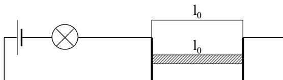
Obr. 16. Uspořádání k paradoxu žárovky.
