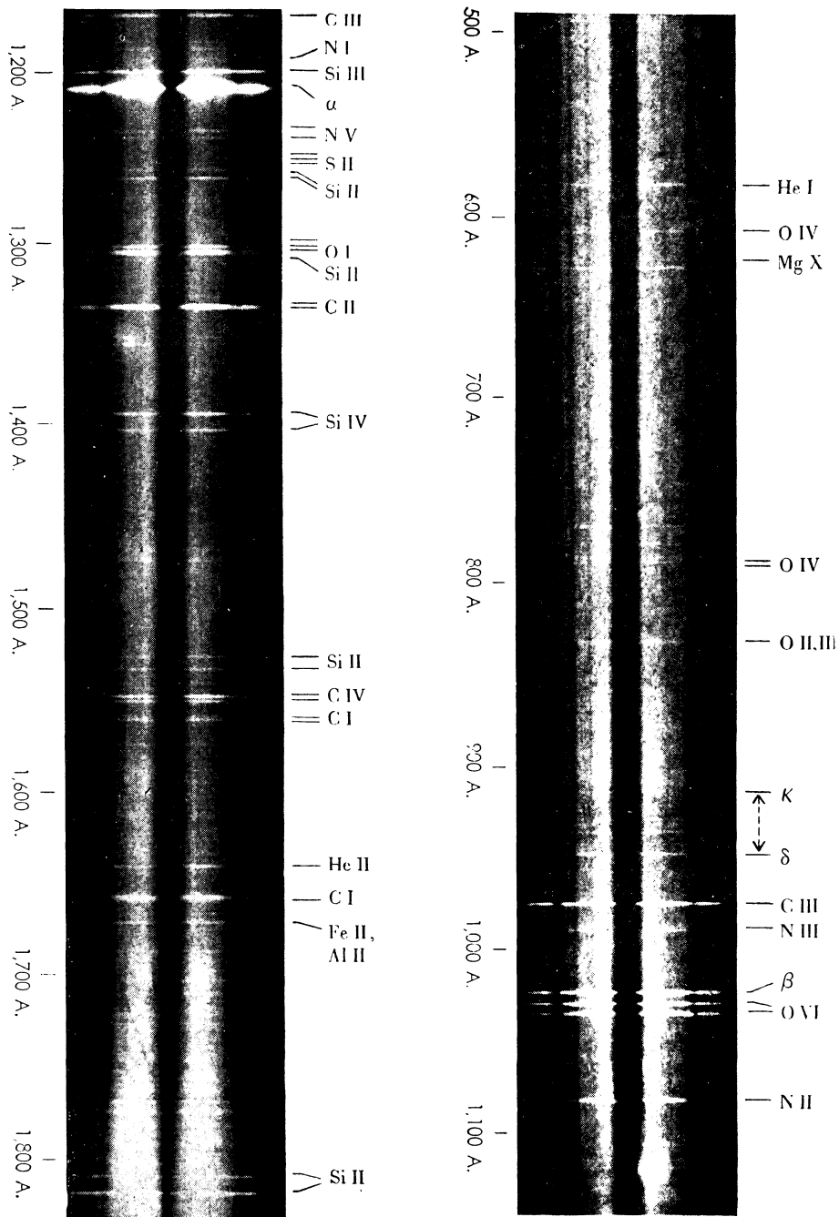
Obr. 1. Spektrum Slunce v ultrafialovém oboru. Řecká písmena označují čáry Lymanovy serie vodíku.
