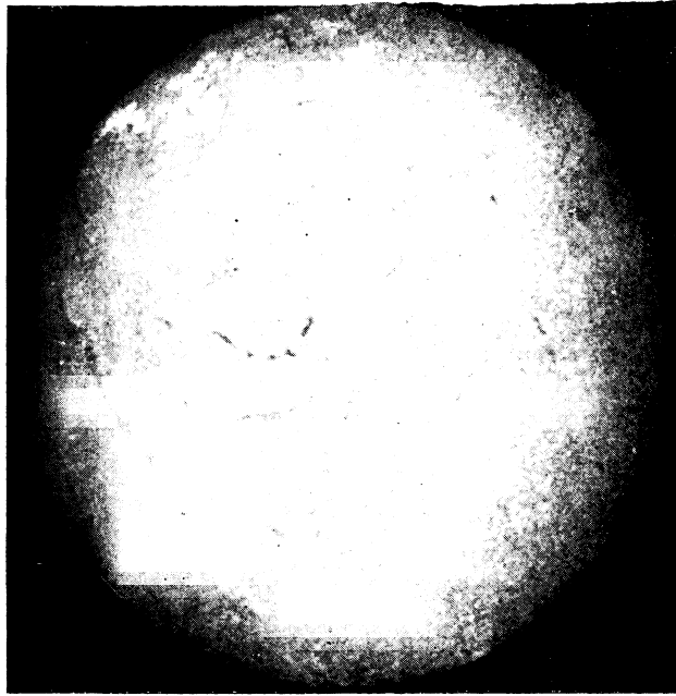
Obr. 2. Monochromatické snímky Slunce ve spektrální čáře L_{\alpha} (vlevo) a H_{\alpha} (vpravo).
