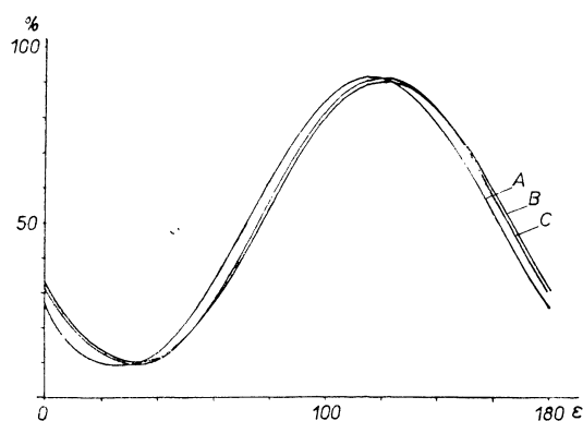
Obr. 8. Priebeh jasnosti polarizačných farieb pre normály A, B, C.
