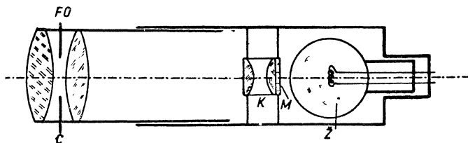
Obr. 6. Schéma osvetľovacieho zariadenia. FO – fotografický objektív, C – clonka, K – kondenzor, M – matnica, Z – žiarovka.
