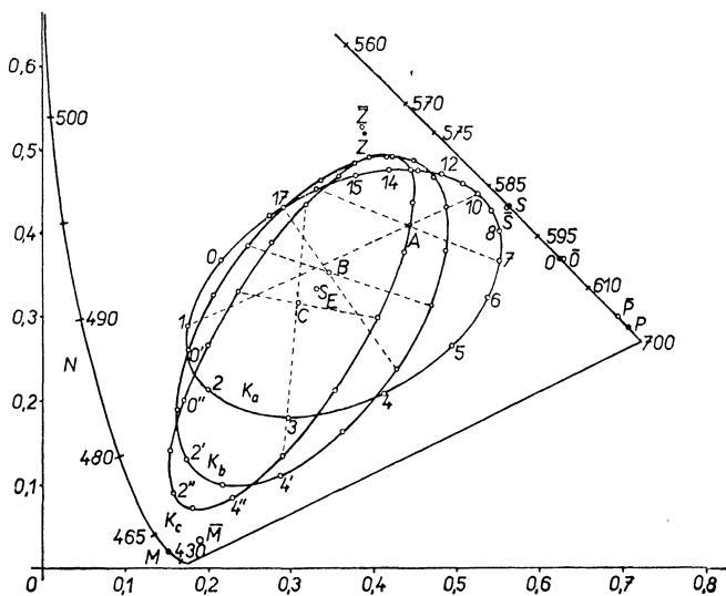
Obr. 4. Polarizačné farby v trojuholníkovom diagrame farieb. Farby P, O, \dots sú teoretické a \bar{P}, \bar{O}, \dots namerané.
