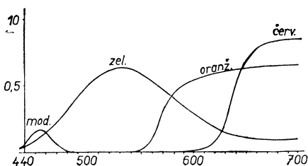
Obr. 7. Krivky priepustnosti kontrolných filtrov.
