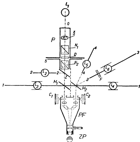
Obr. 5. Schéma experimentálneho zariadenia. Priamky 2 2 atď. sú dráhy možného posuvu príslušných zdrojov.
