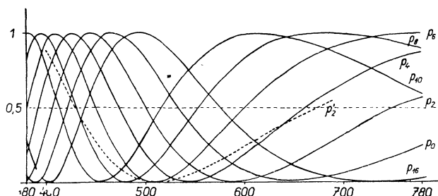
Obr. 2. Krivky priepustnosti. Krivka p platí pre kremennú dosičku o hrúbke 3,39 mm.
