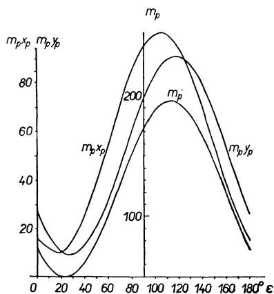
Obr. 3. Grafická závislosť trichromatických súradníc a modulu polarizačných farieb od skríženia nikolov \epsilon .
